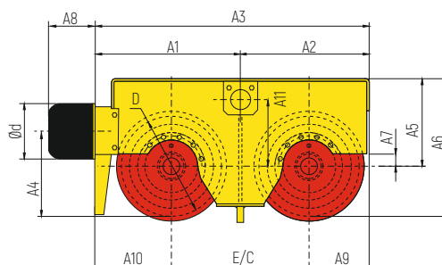
Тележка Ø 500 - 630
