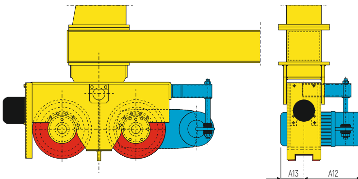
Тележка Ø 315 - 400
